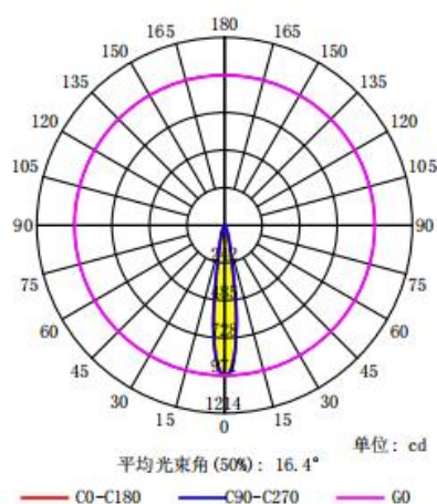
配光曲线
